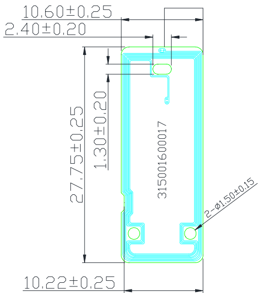
FPCB面
